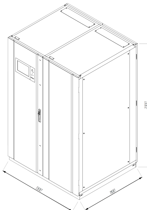
Рис. 3-2-6 Габариты ИБП 400кВА и 500кВА
