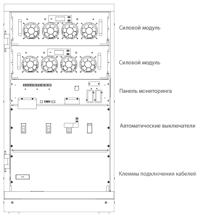
Рис. 2-8-3 Внешний вид 80 кВА и 100 кВА
