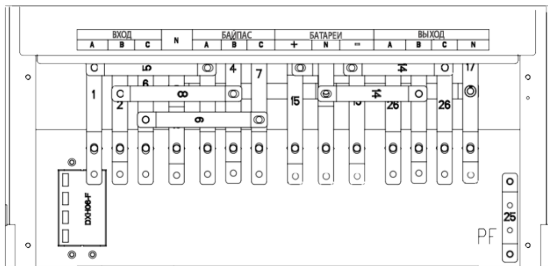
Рис. 3-11-1 Подключение кабелей к ИБП 60 кВА, 90 кВА и 120 кВА
