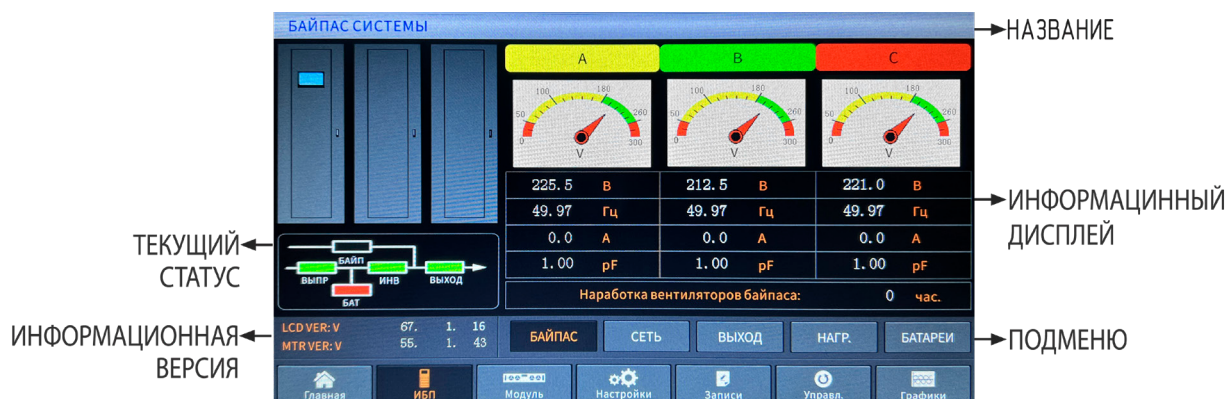
Рис. 4 -4. Меню ИБП
