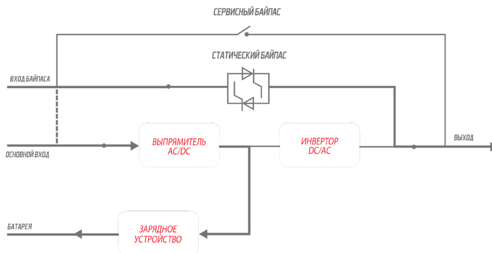
Рис. 2-7 ECO режим
