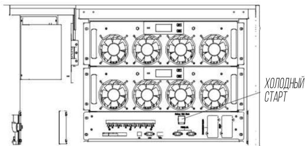
Рис. 4-1. Холодный старт.
