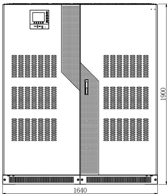
Вид спереди
